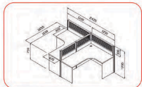
MT-WS012C 2455(W) x 1655(D) x 1200(H) mm.
