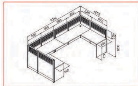
MT-WS022 3310(W) x 1655(D) x 1200(H) mm.
