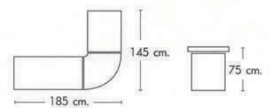
CARIVER SET W185 x D145 x H75 cm.
