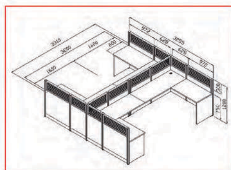
MT-WS024 3310(W) x 3255(D) x 1200(H) mm.
