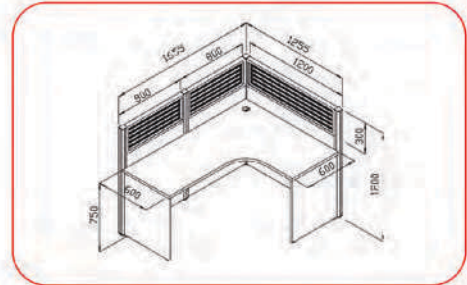
MT-WS011C 1655(W) x 1255(D) x 1200(H) mm.
